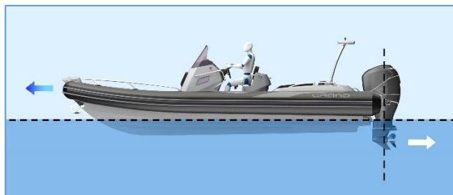
Fig. 22. Optimum trim.
